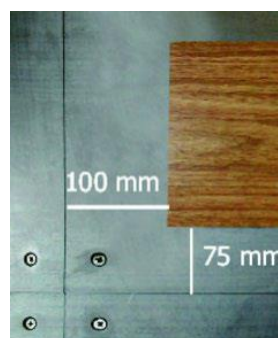
Positie van een tegel van het formaat 1000 x 150 mm. De afstand van de rand van een paneel van een systeemvloer dient in de lengte 75 mm en aan de kopse kant 100 mm te bedragen.
