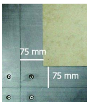
Positie van een tegel van het formaat 450 x 450 mm, de afstand van de rand van een paneel van een systeemvloer dient aan alle zijden 75 mm te bedragen.
